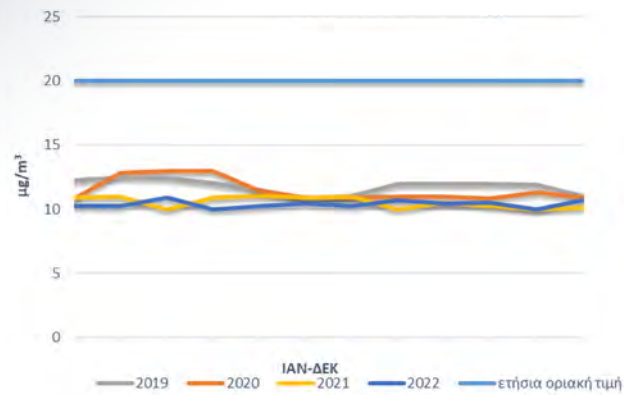
Μέσες Μηνιαίες Συγκεντρώσεις PM 2.5
