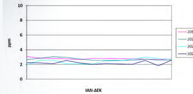
Μέσες Μηνιαίες Συγκεντρώσεις CH 4
