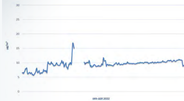
Μέσες Ημερήσιες Συγκεντρώσεις H 2 S - Σταθμός AVIN
