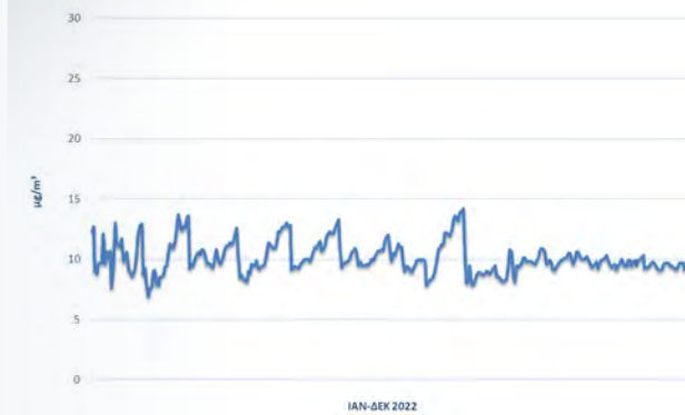
Μέσες Ημερήσιες Συγκεντρώσεις H 2 S - Σταθμός T752
