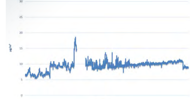
Μέσες Ωριαίες Συγκεντρώσεις H 2 S - Σταθμός AVIN
