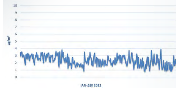
Μέσες Ημερήσιες Συγκεντρώσεις Βενζολίου
