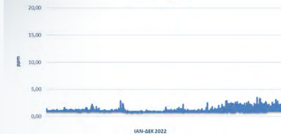
Μέσες Ωριαίες Συγκεντρώσεις NMHC
