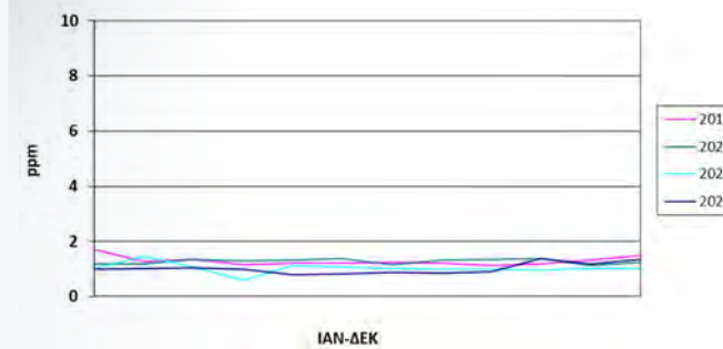
Μέσες Μηνιαίες Συγκεντρώσεις NMHC
