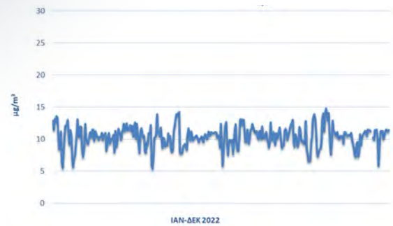
Μέσες Ημερήσιες Συγκεντρώσεις PM 2.5
