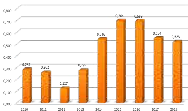
Ποσότητα Στερεών Αποβλήτων ανά πρώτες ύλες (ΜΤ/χιλ. ΜΤ)
